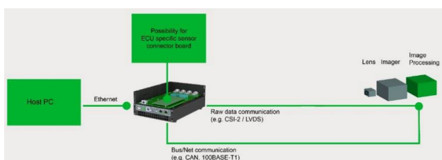
图4：b-HiL示意图
